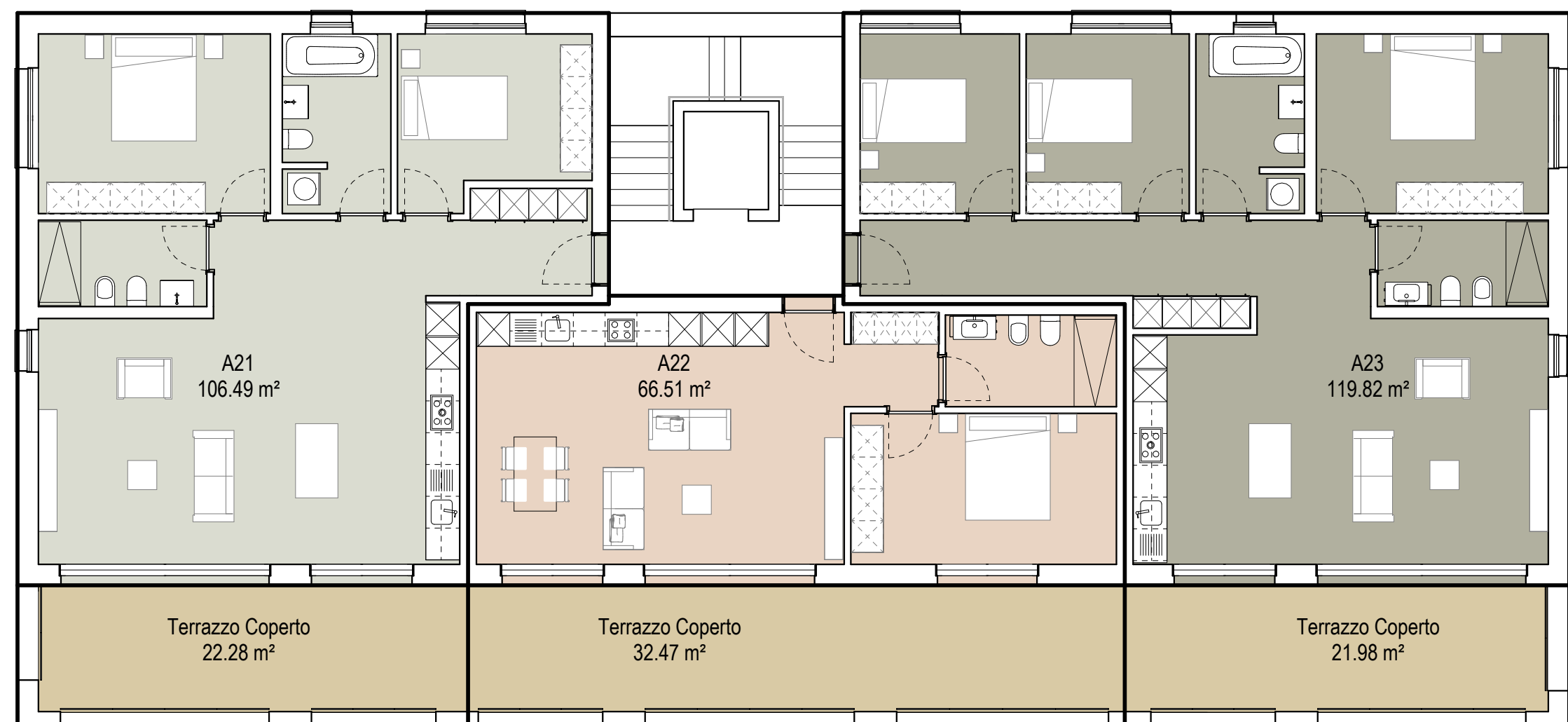
R - Piano Secondo 1:100
